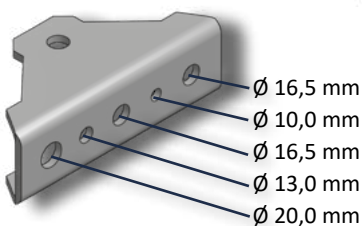
Lochbild Endgelenk
